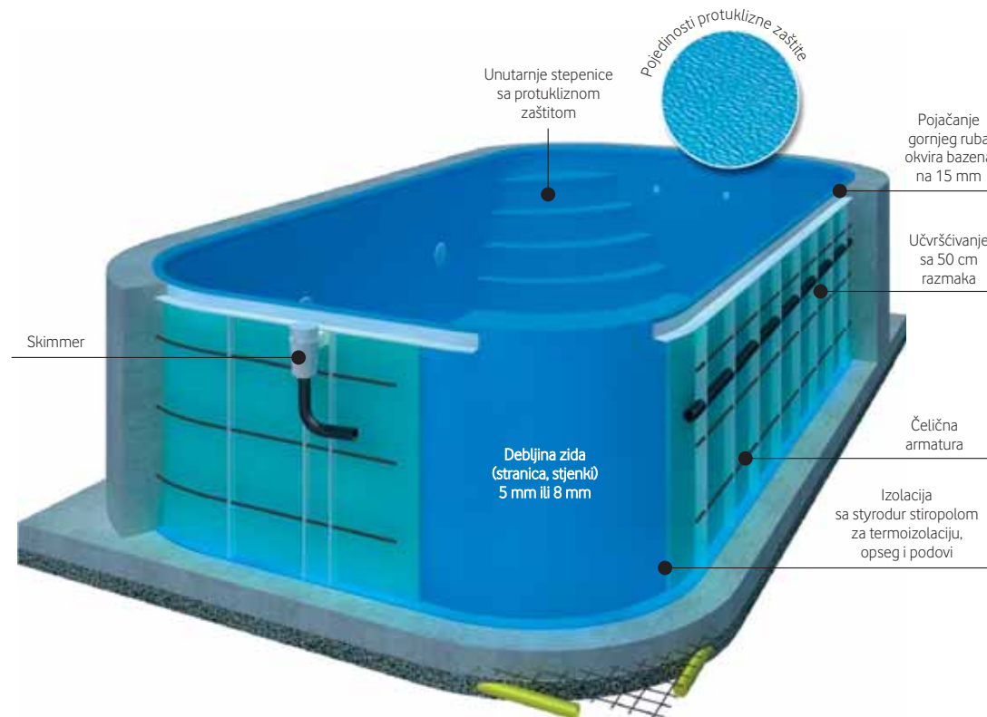
Skimmer bazen sa ugrađenim unutrašnjim stepenicama
